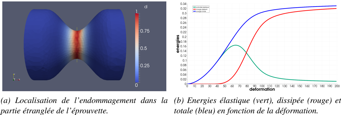
FIGURE 3 – Rupture d'une éprouvette diablo soumise à un essai de traction. Simulation 3D réalisée avec le code éléments finis MEF++
